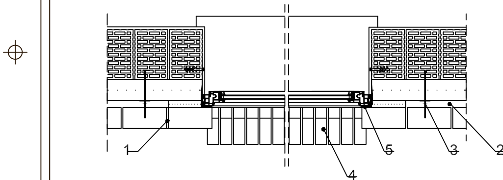
Przekrój A-A
